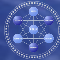
STAR PERLE
