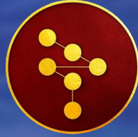
VENUS
