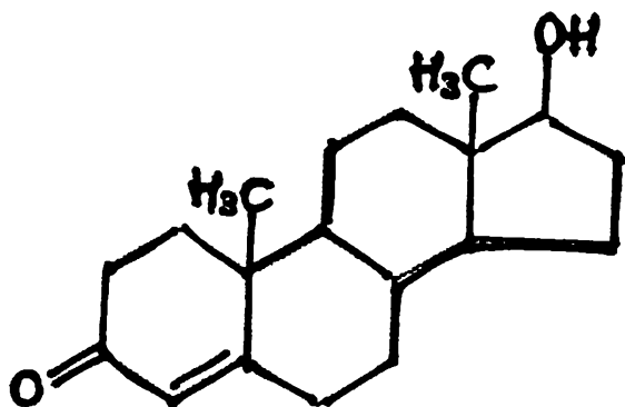
ESTRUCTURA QUÍMICA de la TESTOSTERONA
